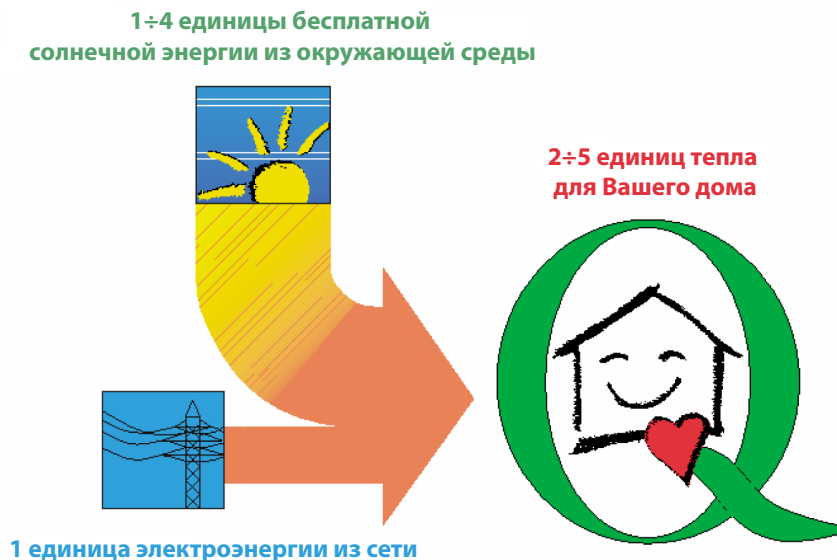
Рис. 2 Принцип действия теплового насоса
